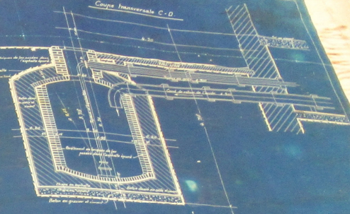
Coupe transversale C-D
