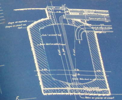
Coupe transversale A-B
