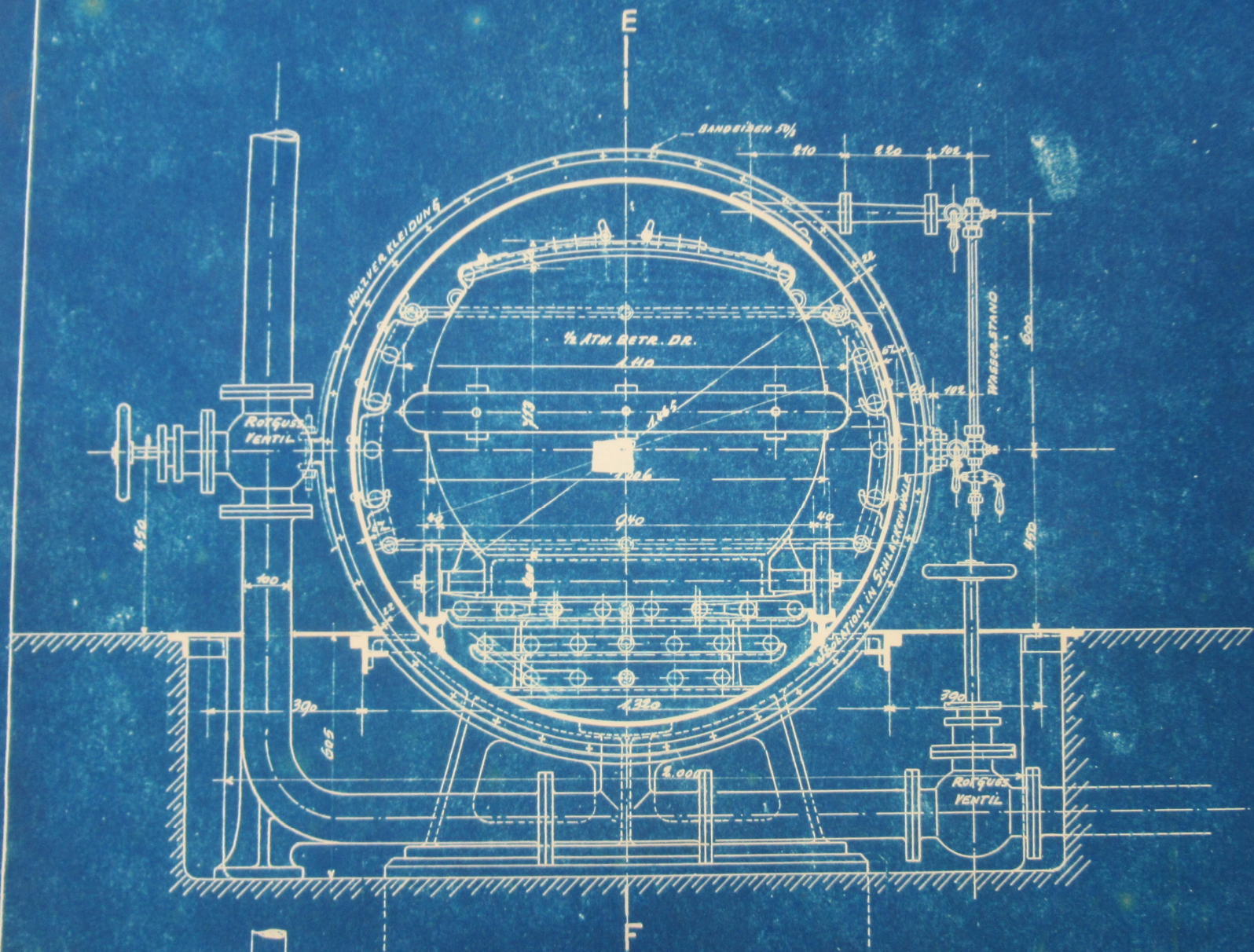
SCHNITT C-D.
