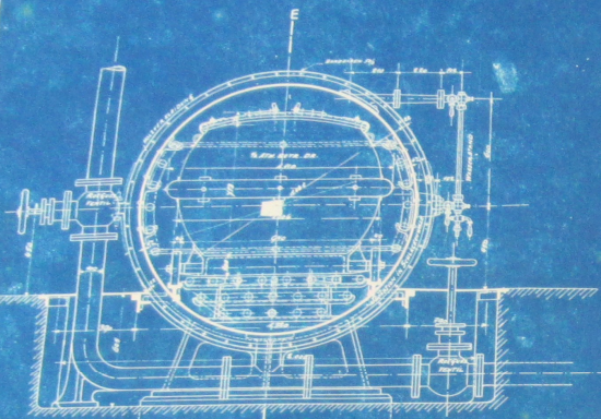
SCHNITT C-D.
