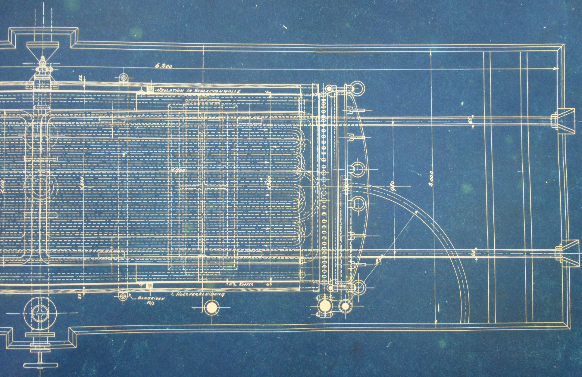
SCHNITT A-B.
