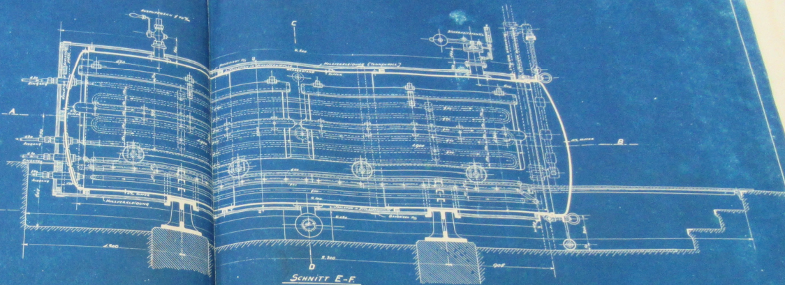
SCHNITT E-F.
