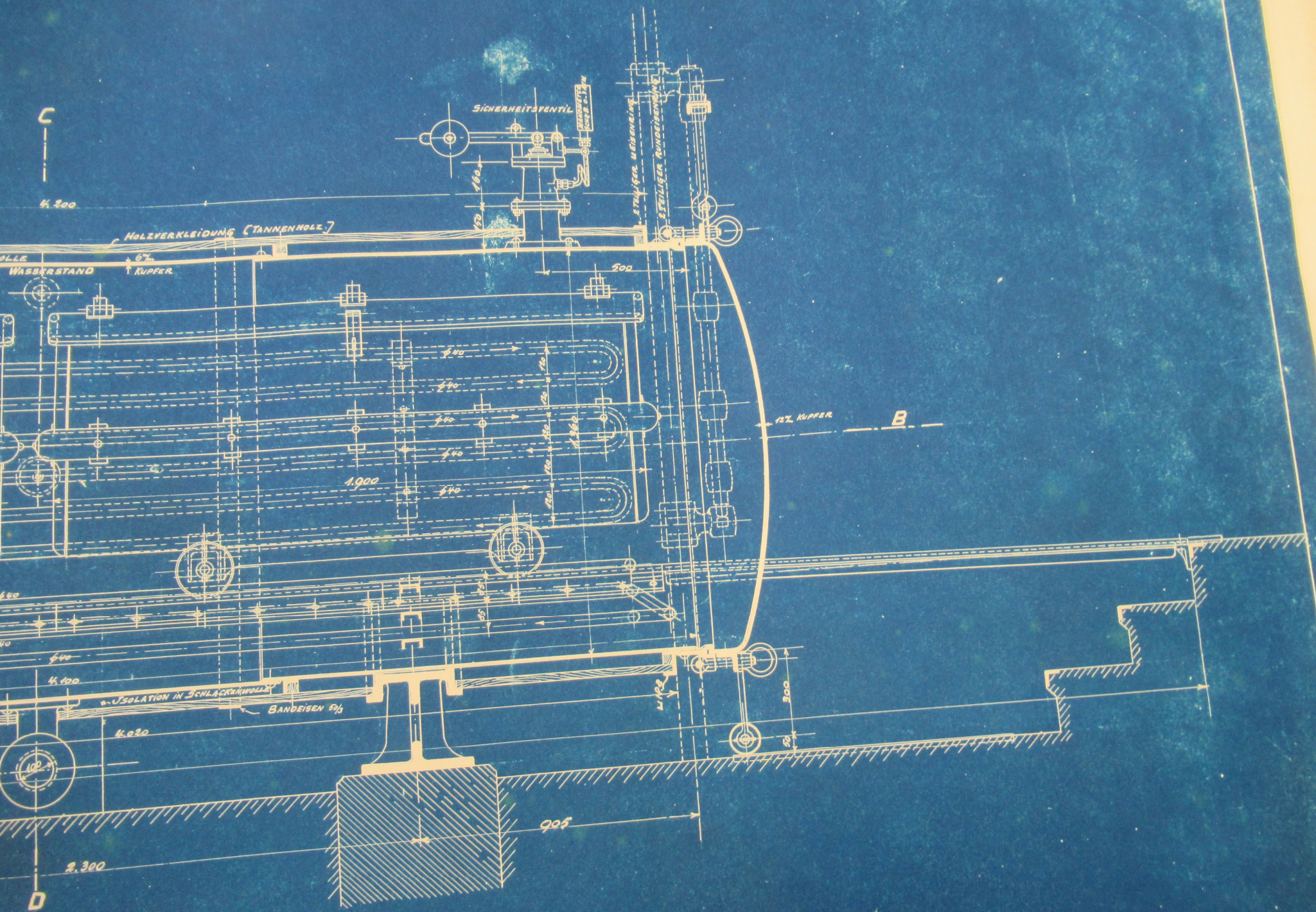
SCHNITT E-F
