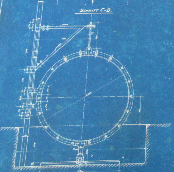
ANSICHT DES DECKELS
