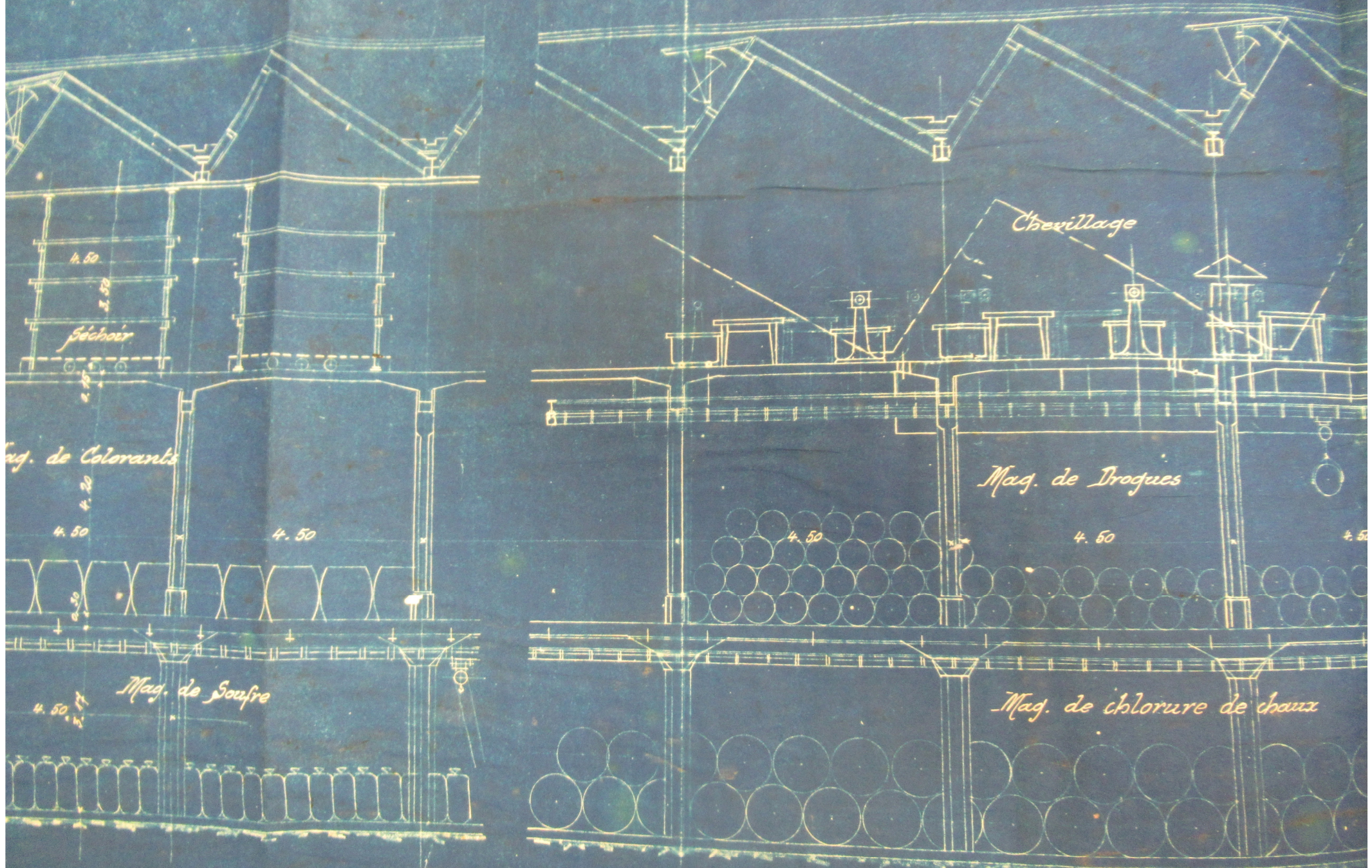
Coupe transversale T-T
