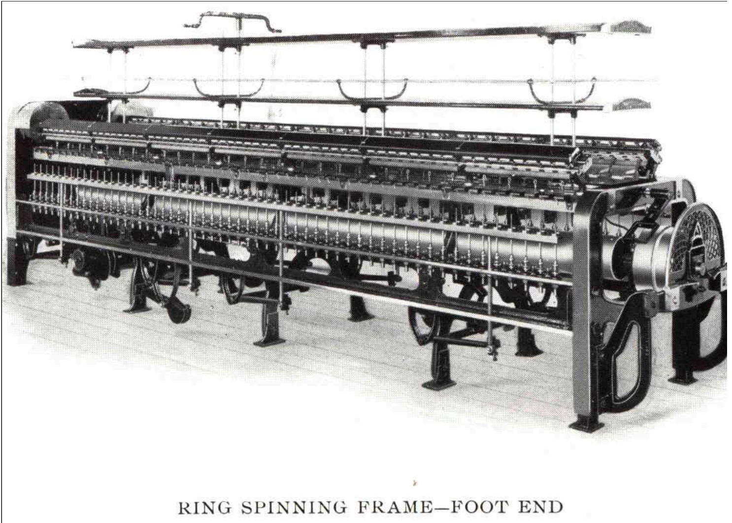
RING SPINNING FRAME-FOOT END
