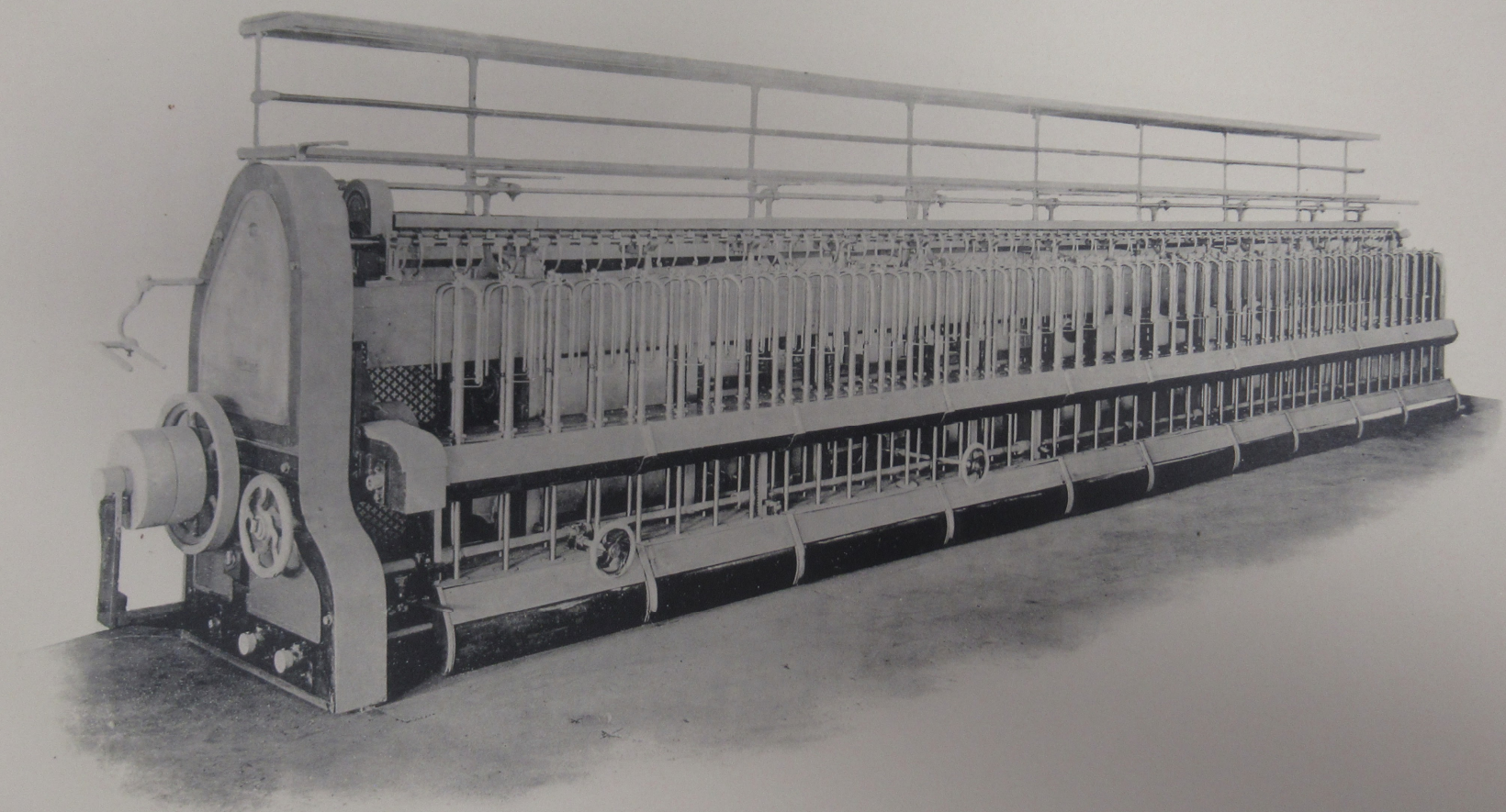
BANC A BROCHES INTERMÉDIAIRE
