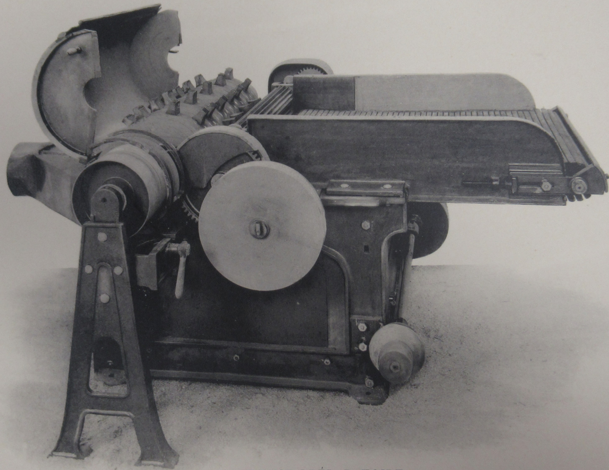
OUVREUSE PRÉPARATOIRE
