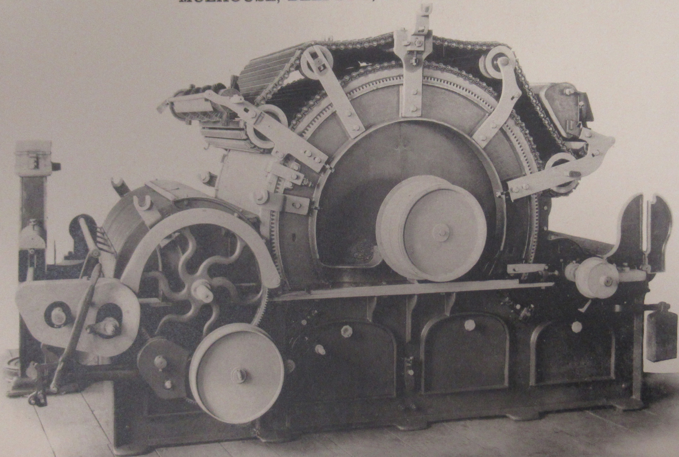
CARDE A CHAPELET (BREVET S. A. C. M.) N° 93
