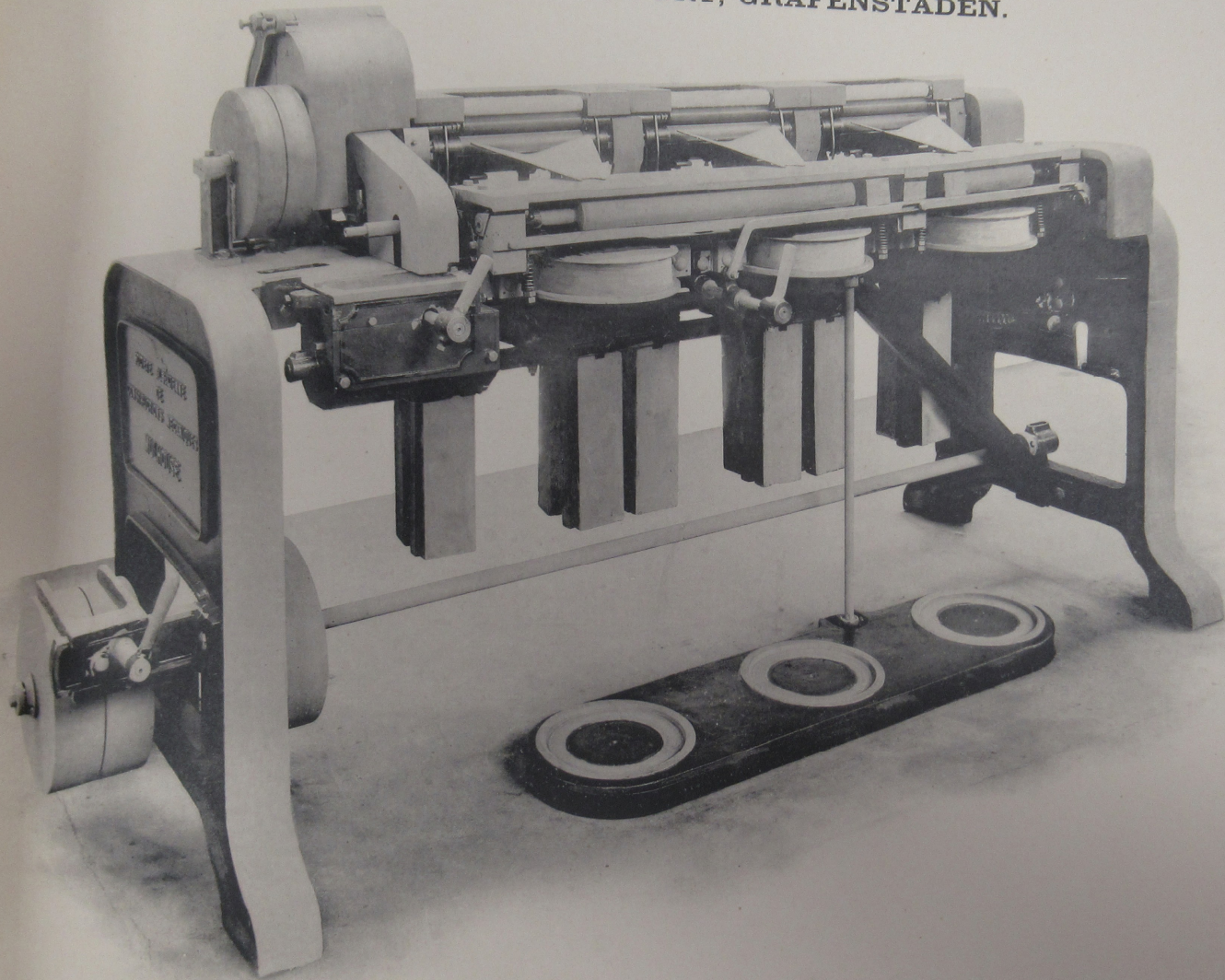
BANC D'ÉTIRAGE A CASSE-MÈCHES ÉLECTRIQUES
