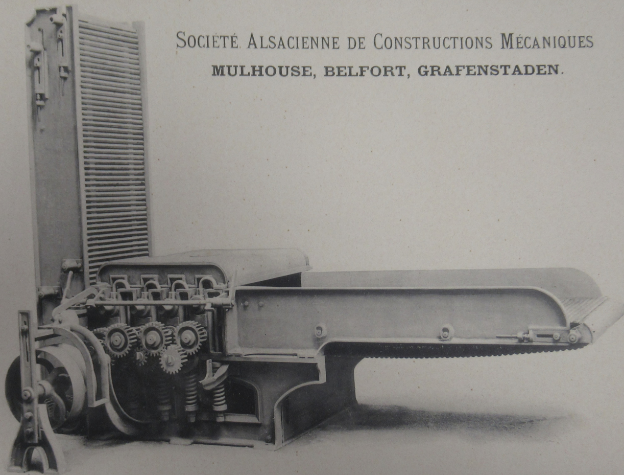
MÉLANGEUSE
