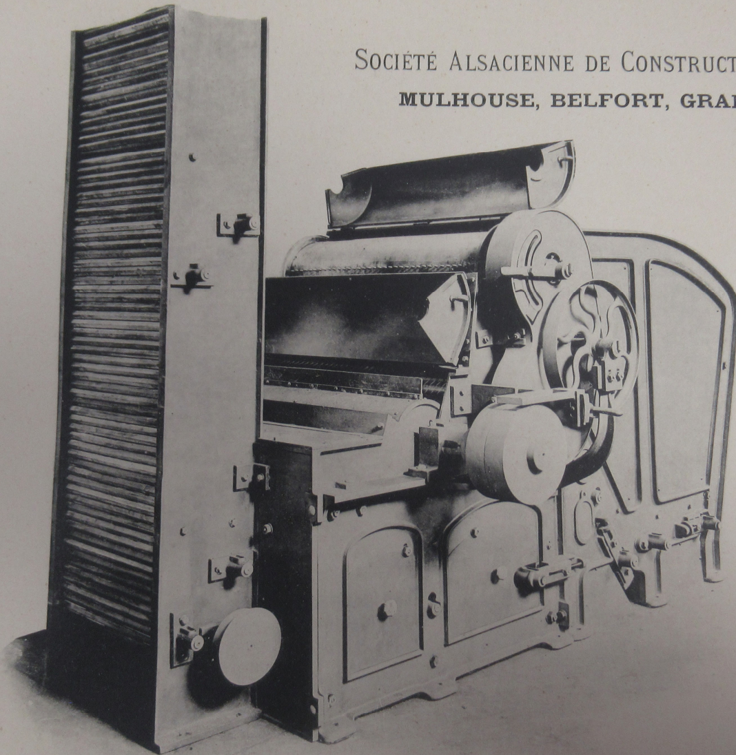
MÉLANGEUSE
