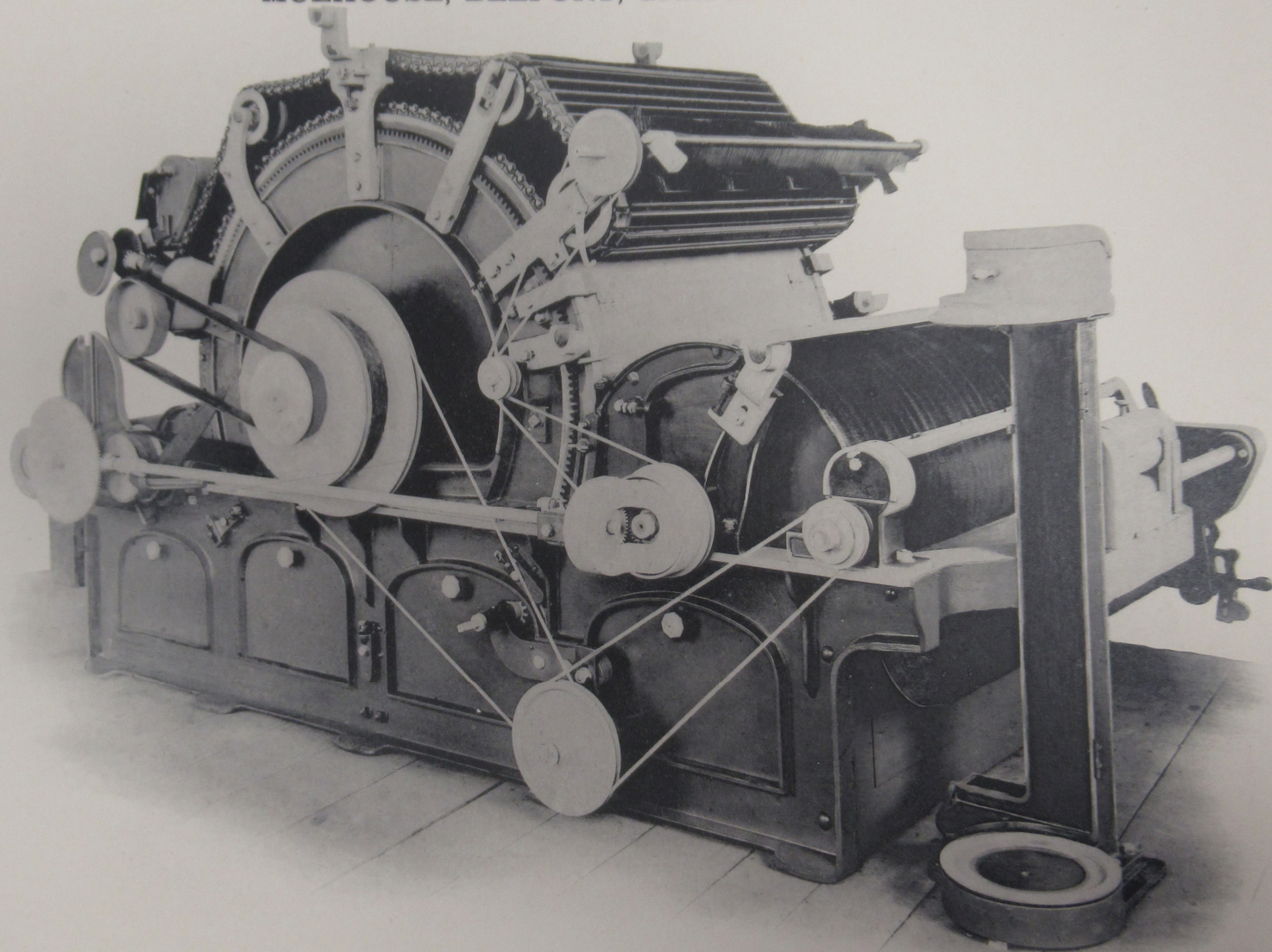
CARDE A CHAPELET (BREVET S. A. C. M.)
