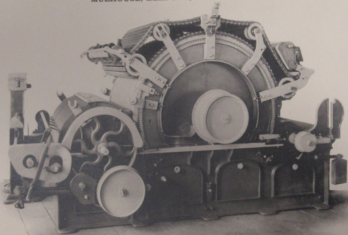
CARDE A CHAPELET (BREVET S. A. C. M.)
