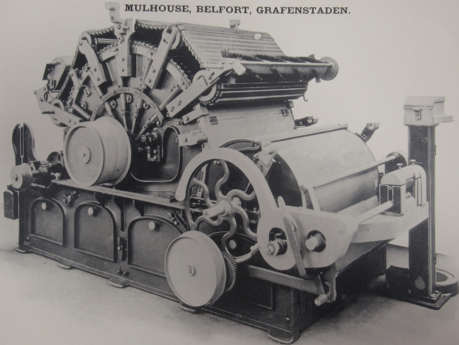
CARDE A CHAPELET (BREVET G. FAUQUET)
