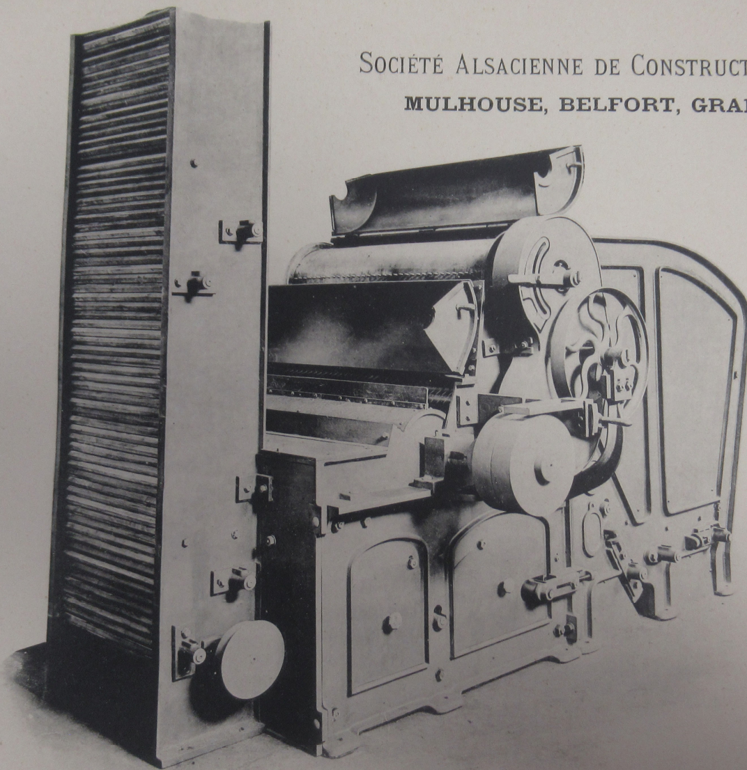
MÉLANGEUSE
