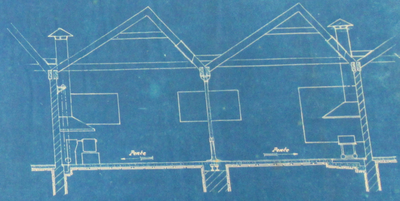
- Coupe E-F -
