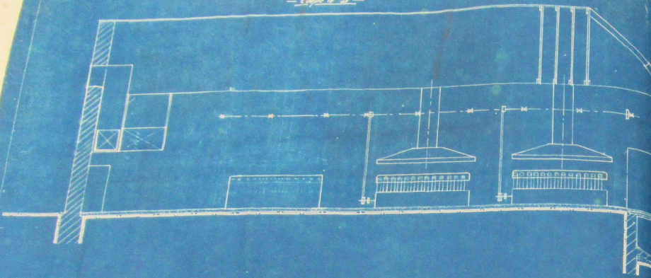
- Coupe A-B -
