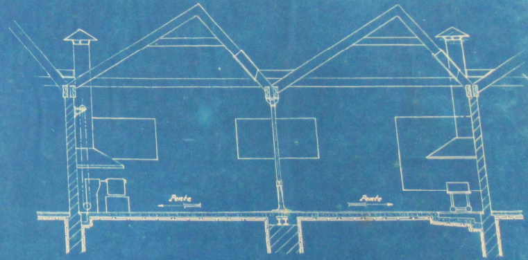
- Coupe E-F -
