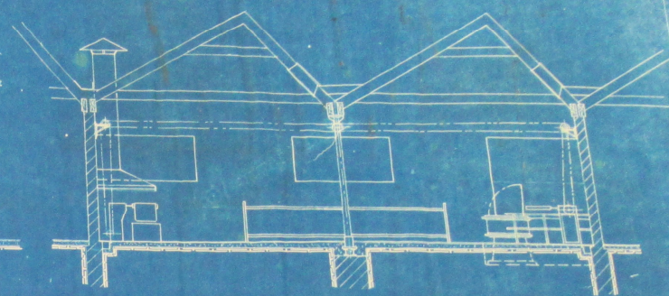
- Coupe E-F -
