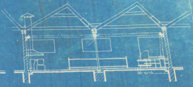
- Coupe E-F -
