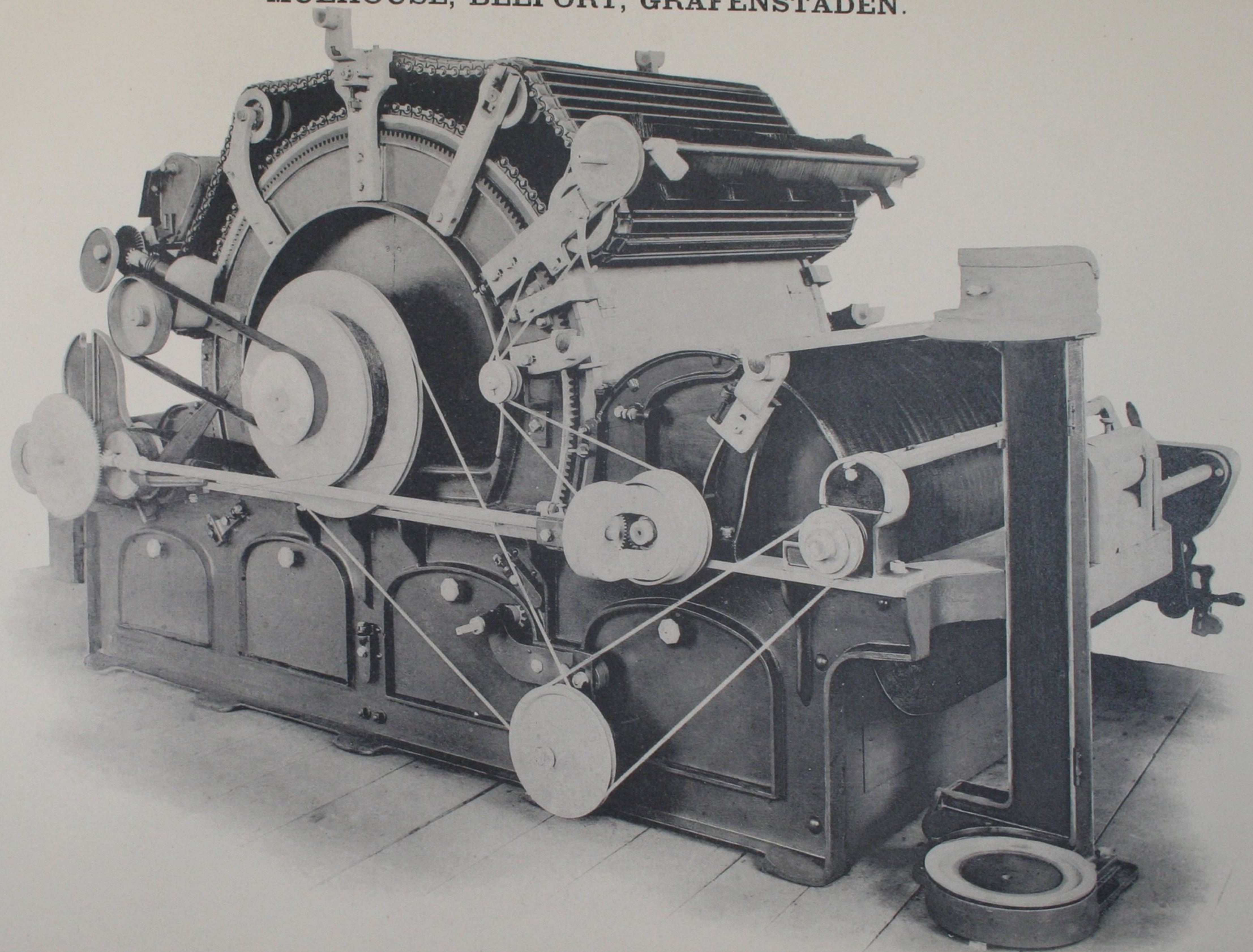
CARDE A CHAPELET (BREVET S. A. C. M.)
