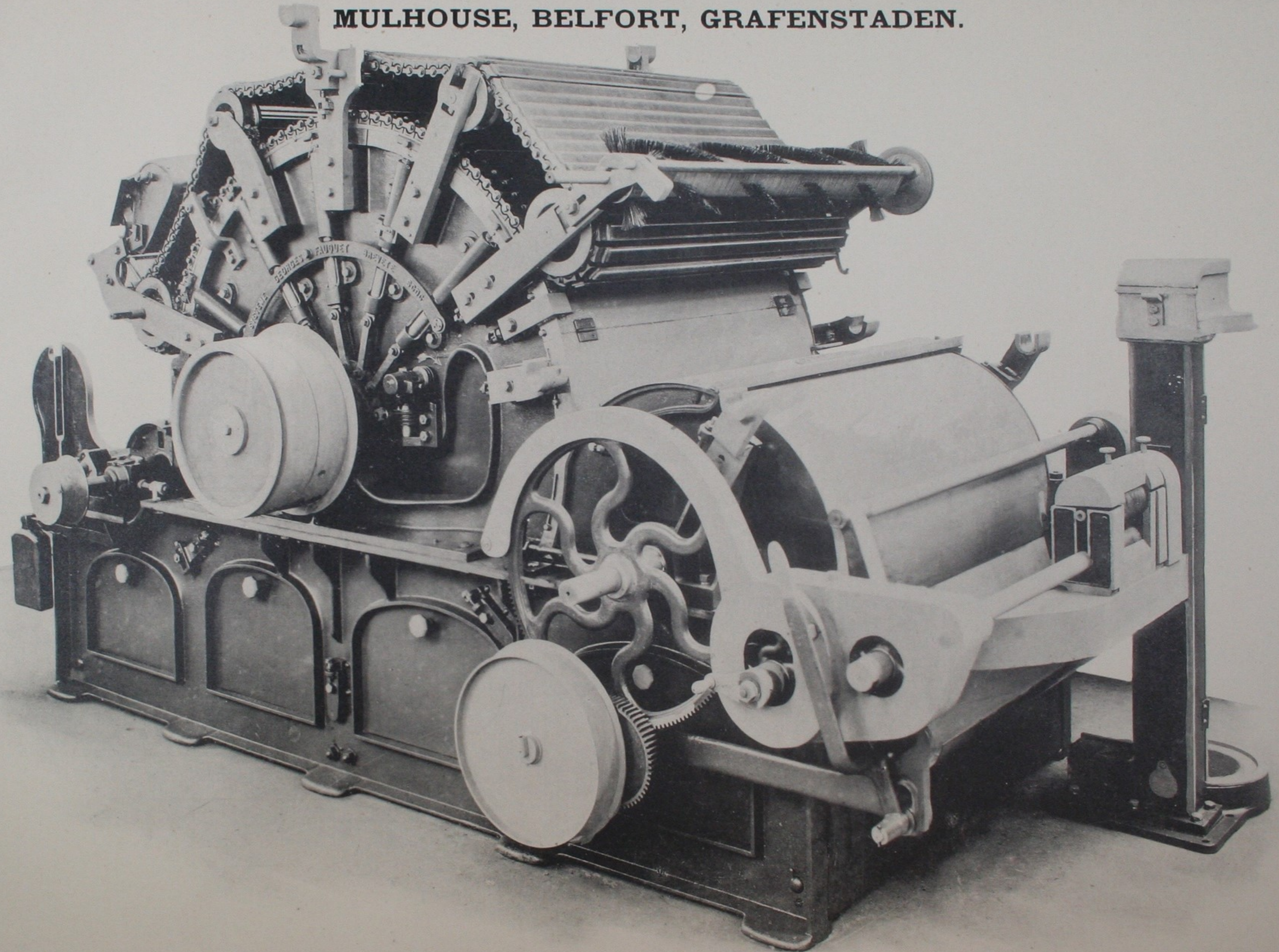
CARDE A CHAPELET (BREVET G. FAUQUET)
