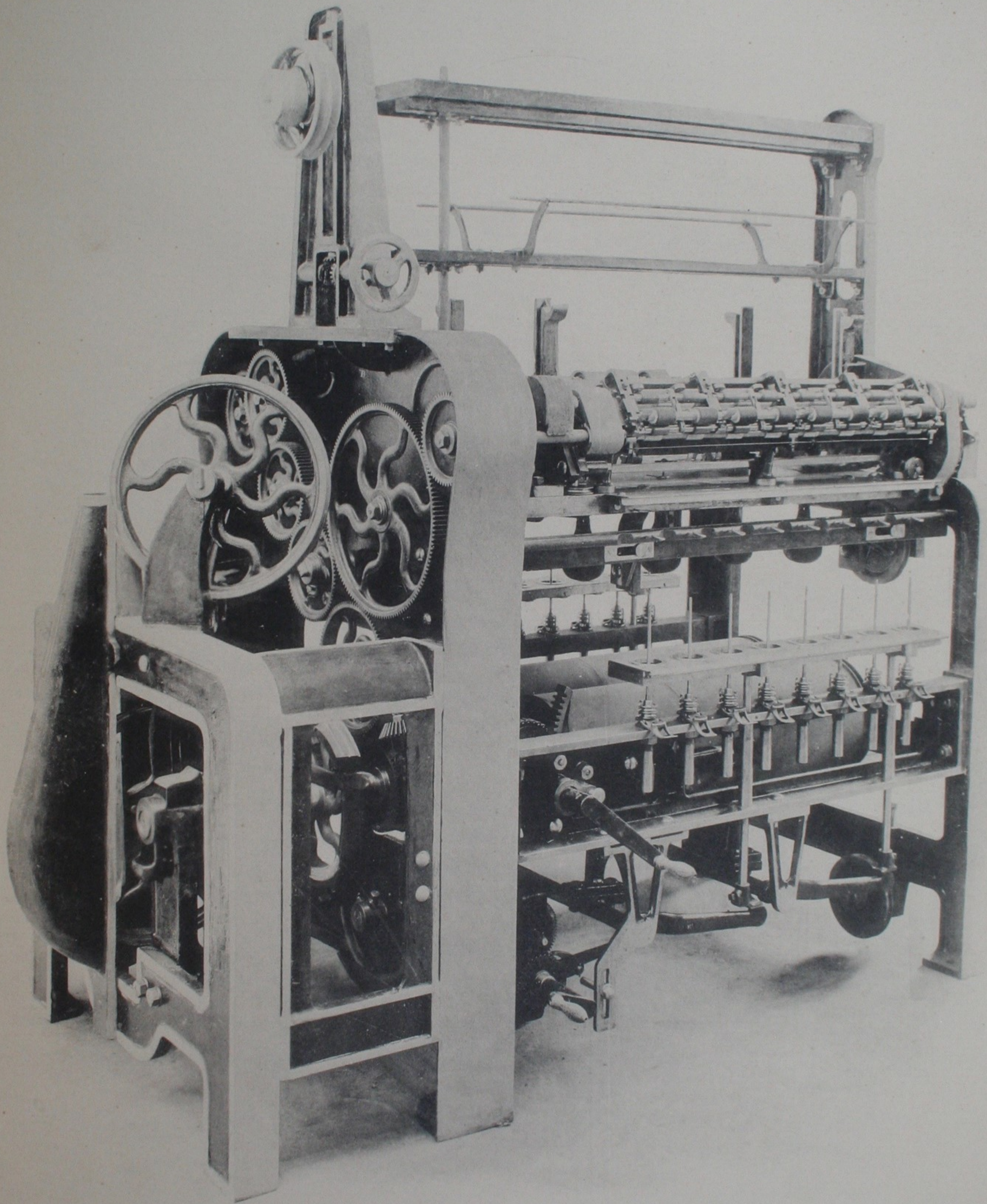
CONTINU A FILER (BREVETS VIMONT-BAZIN)
