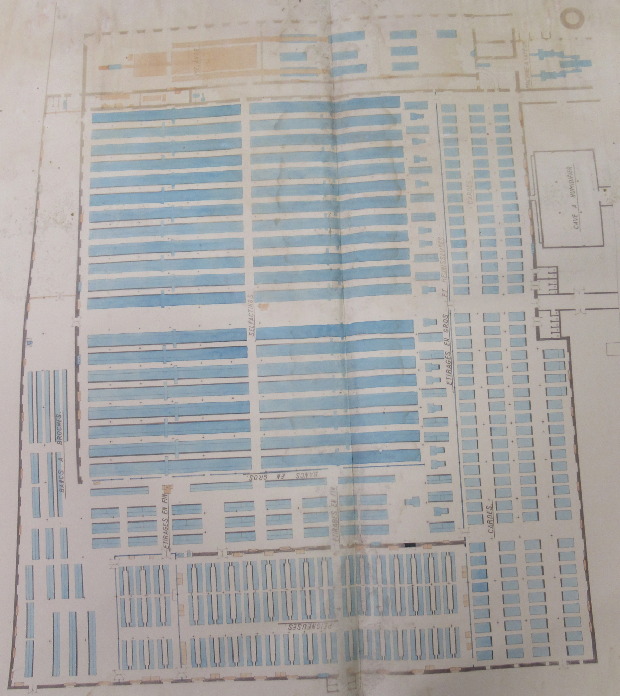
FILATURE A ETAGES
