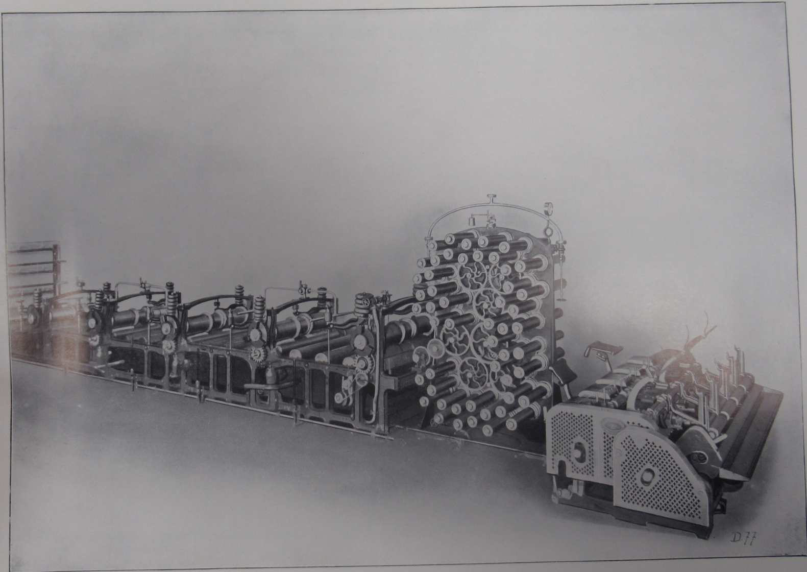
Lisseuse de teinture à 3, 4 ou 5 bains et Intersecting.
