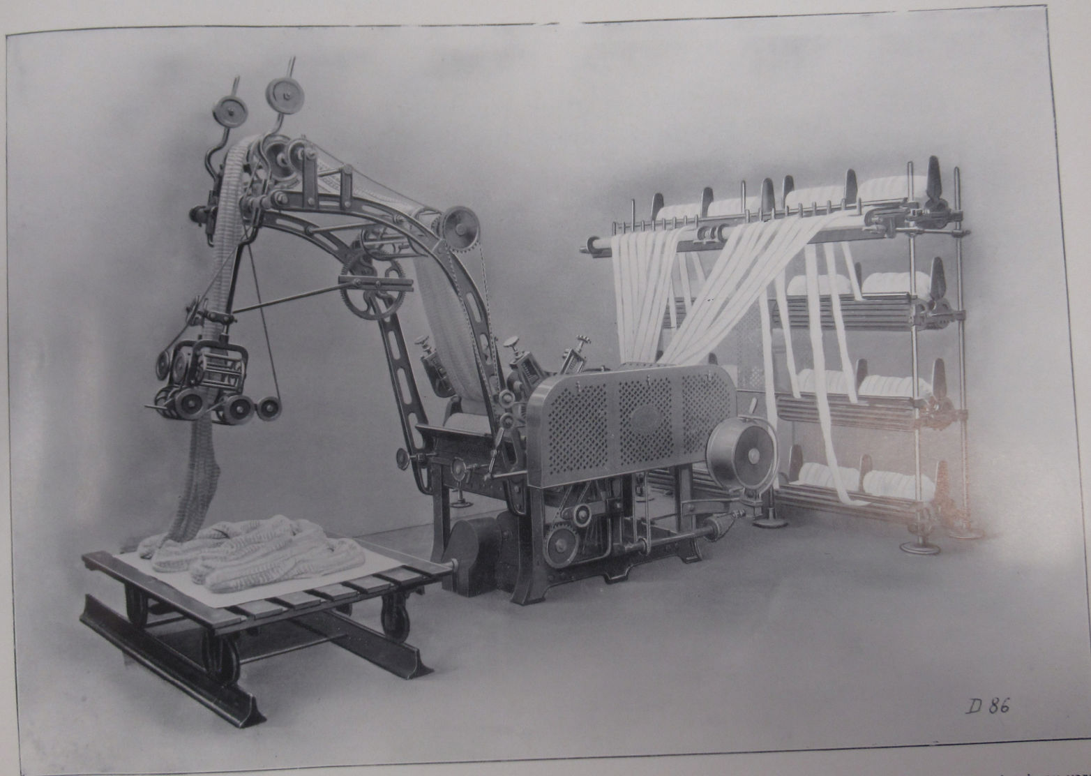
Gillbox pour Vigoureux.
