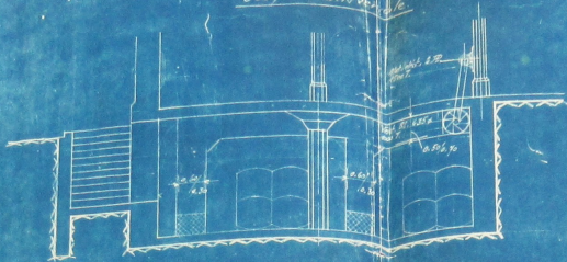
Coupe transversale
