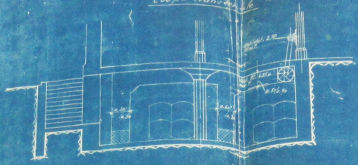
Coupe transverse
