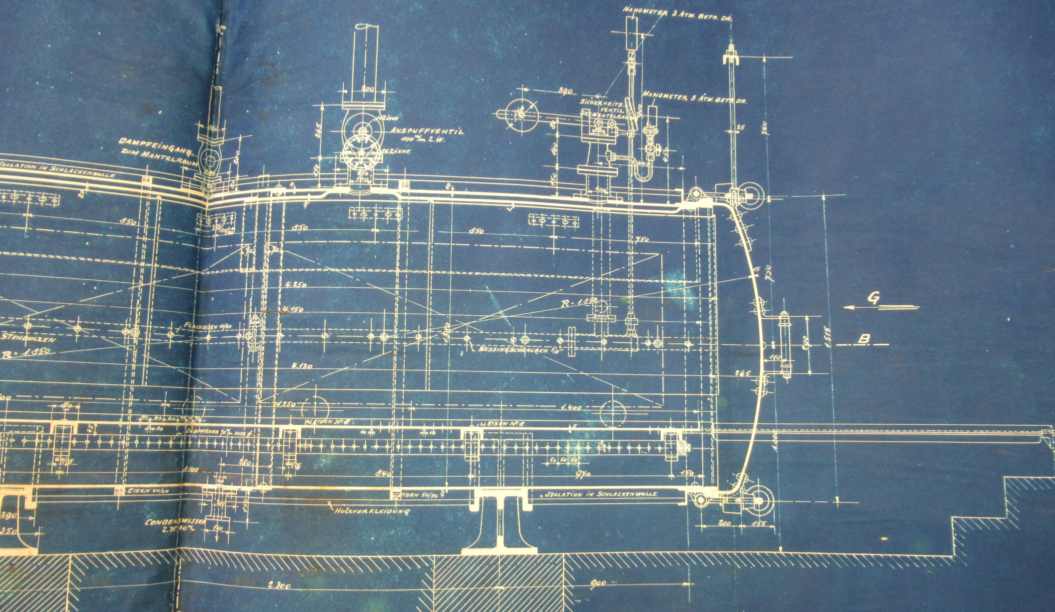
SCHNITT E-F
